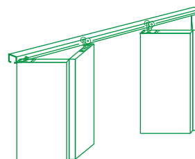
LÙA XẾP 04 CẢNH VỀ 02 BÊN
